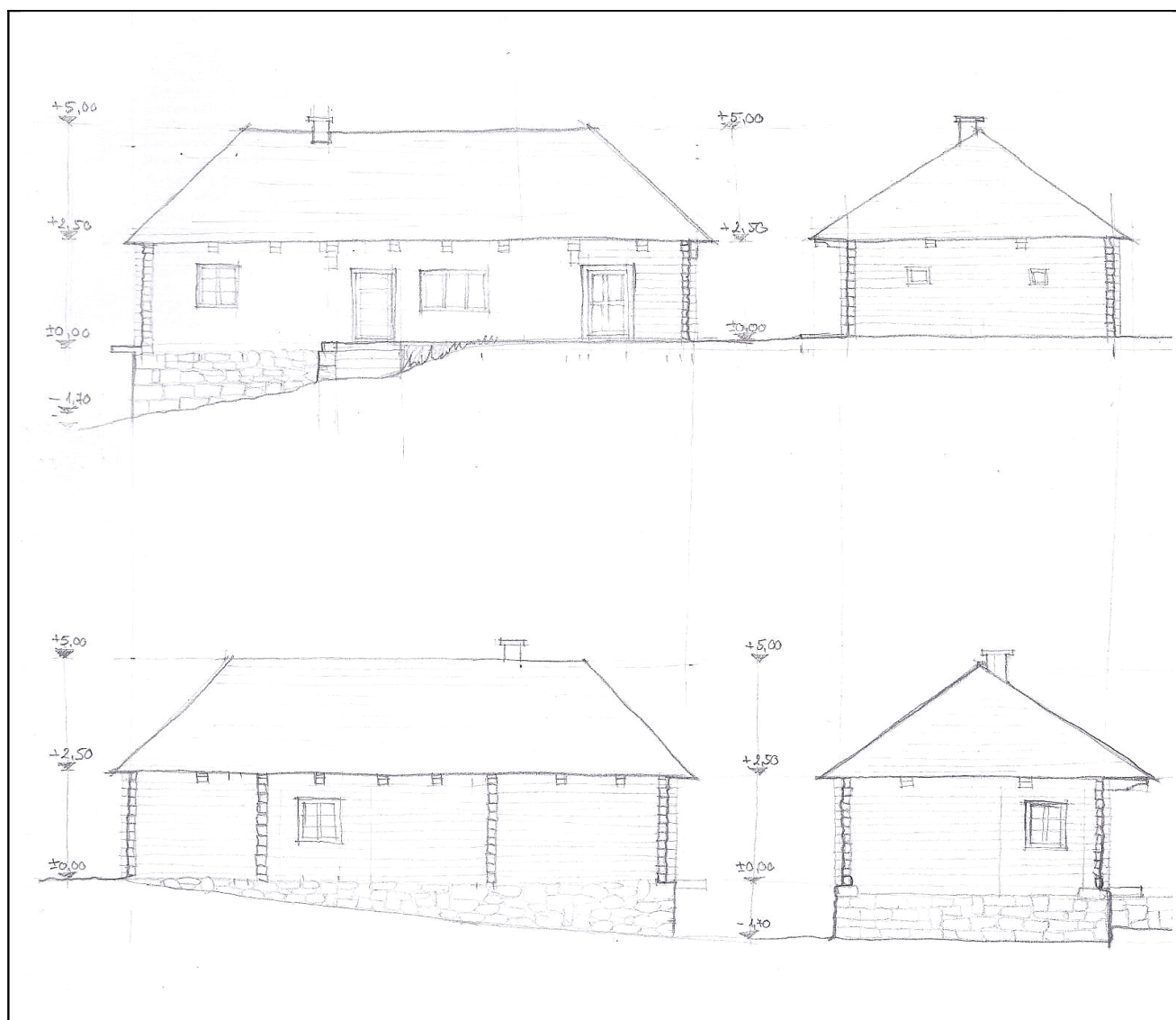
az épület fő méretei, égtájak megjelölése
