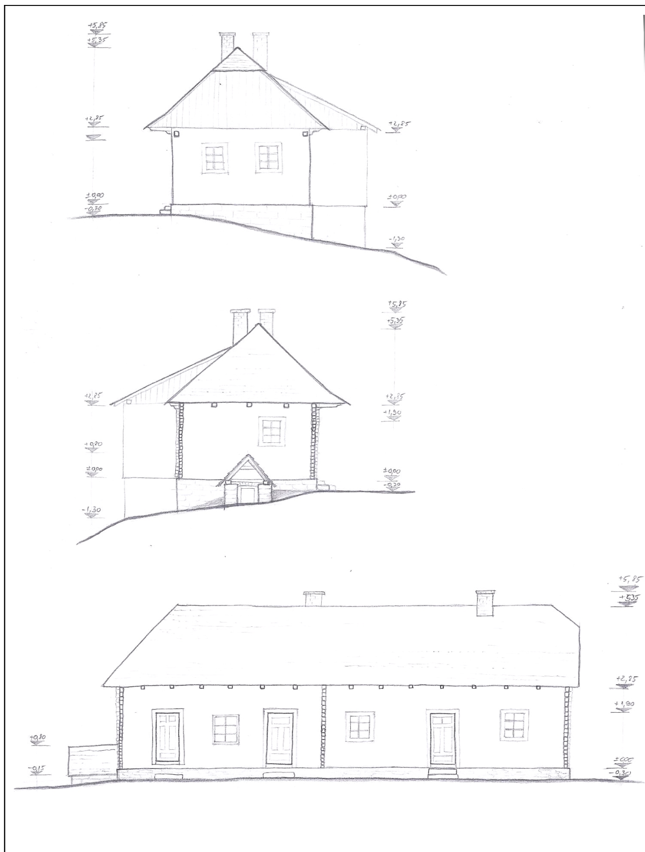
az épület fő méretei, égtájak megjelölése
