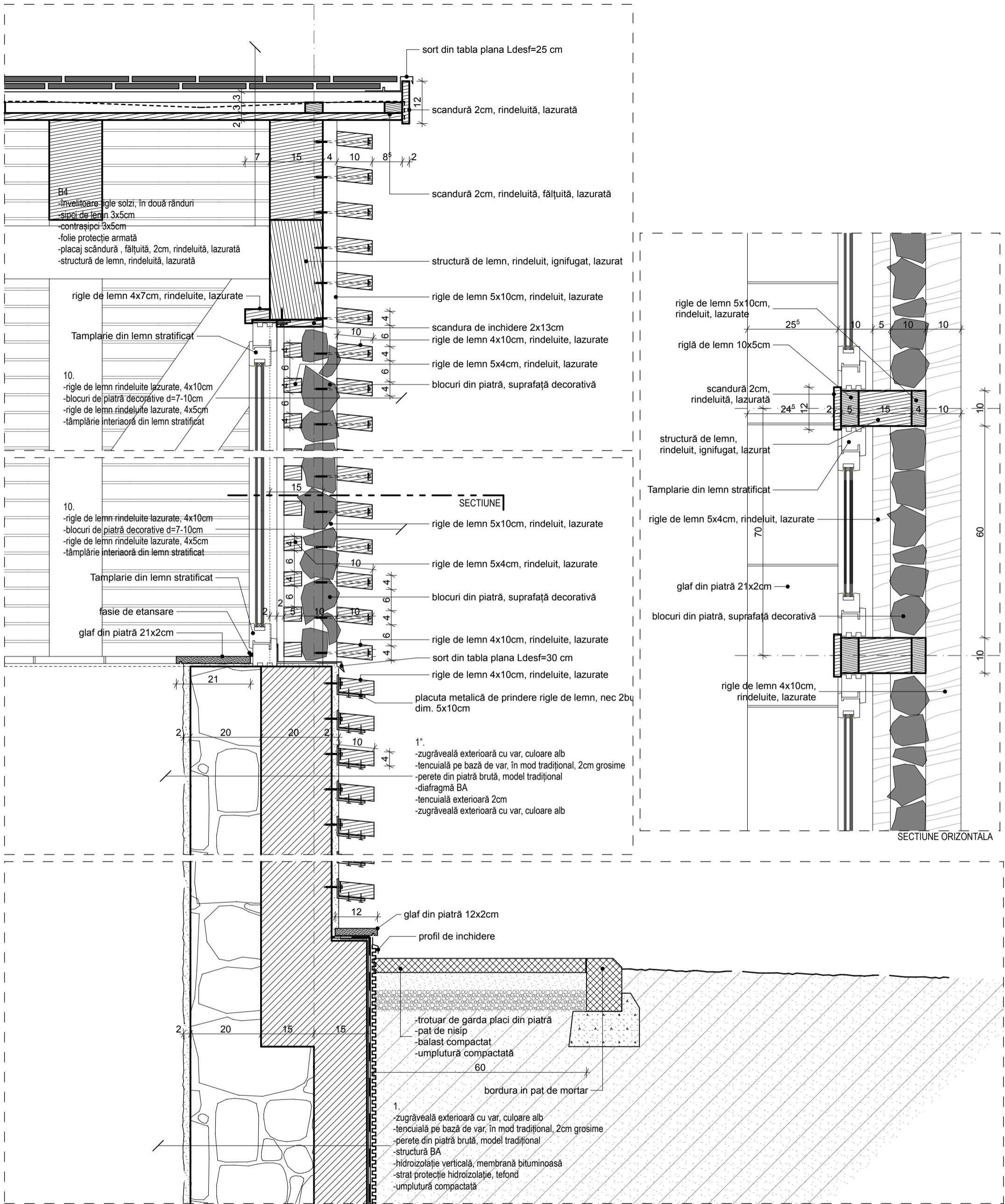
DETALIU APLICABIL LA FRONTOANE SI ZONE CU UMLUTURI COMPACTATE
