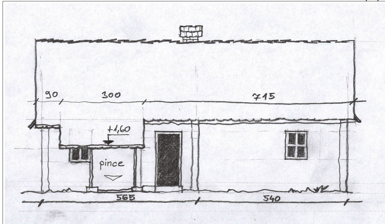
7b. Homlokzati vázlat
