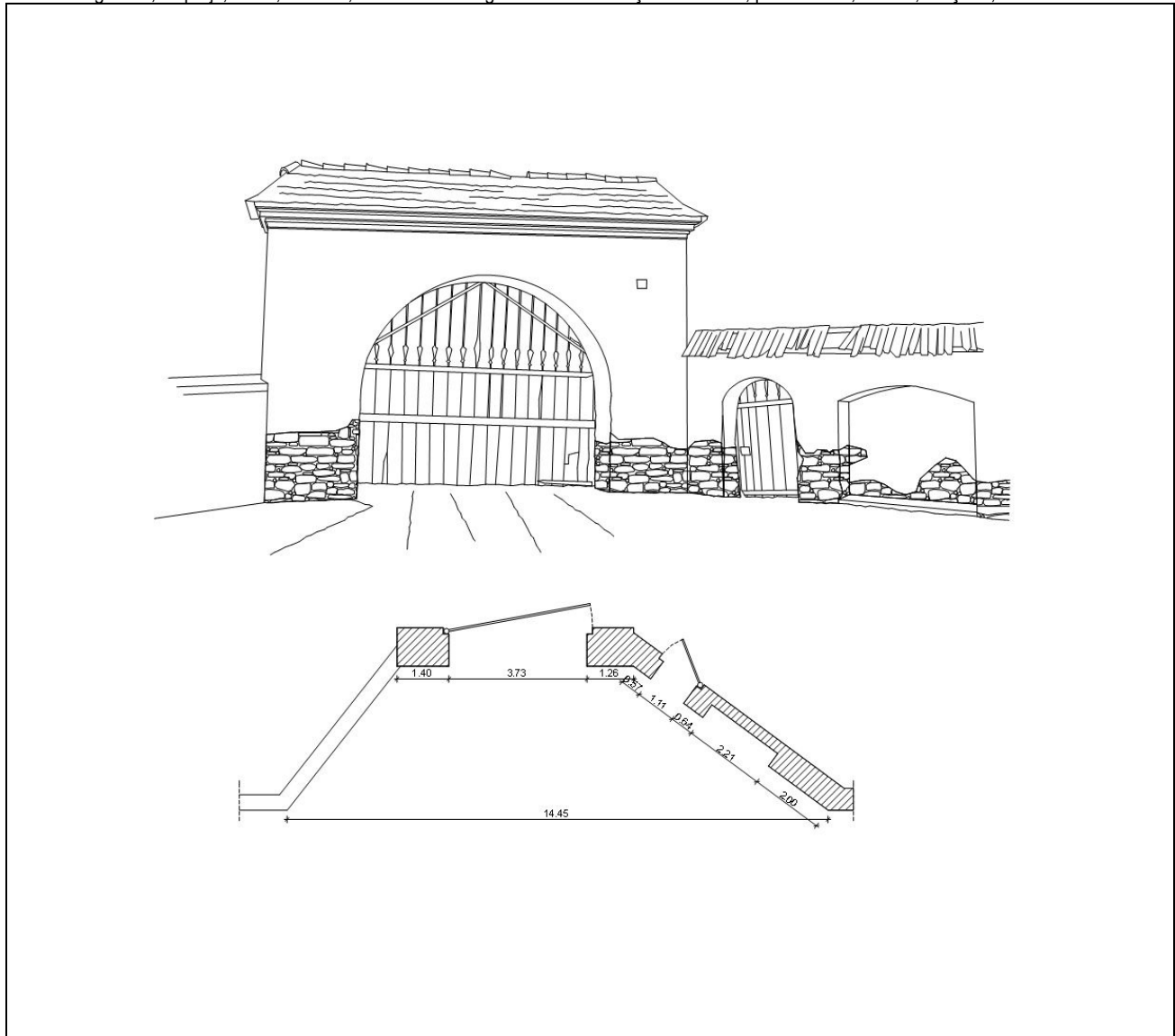
az objektum fő méretei, alaprajzon égtájak, szomszédságok megjelölése
