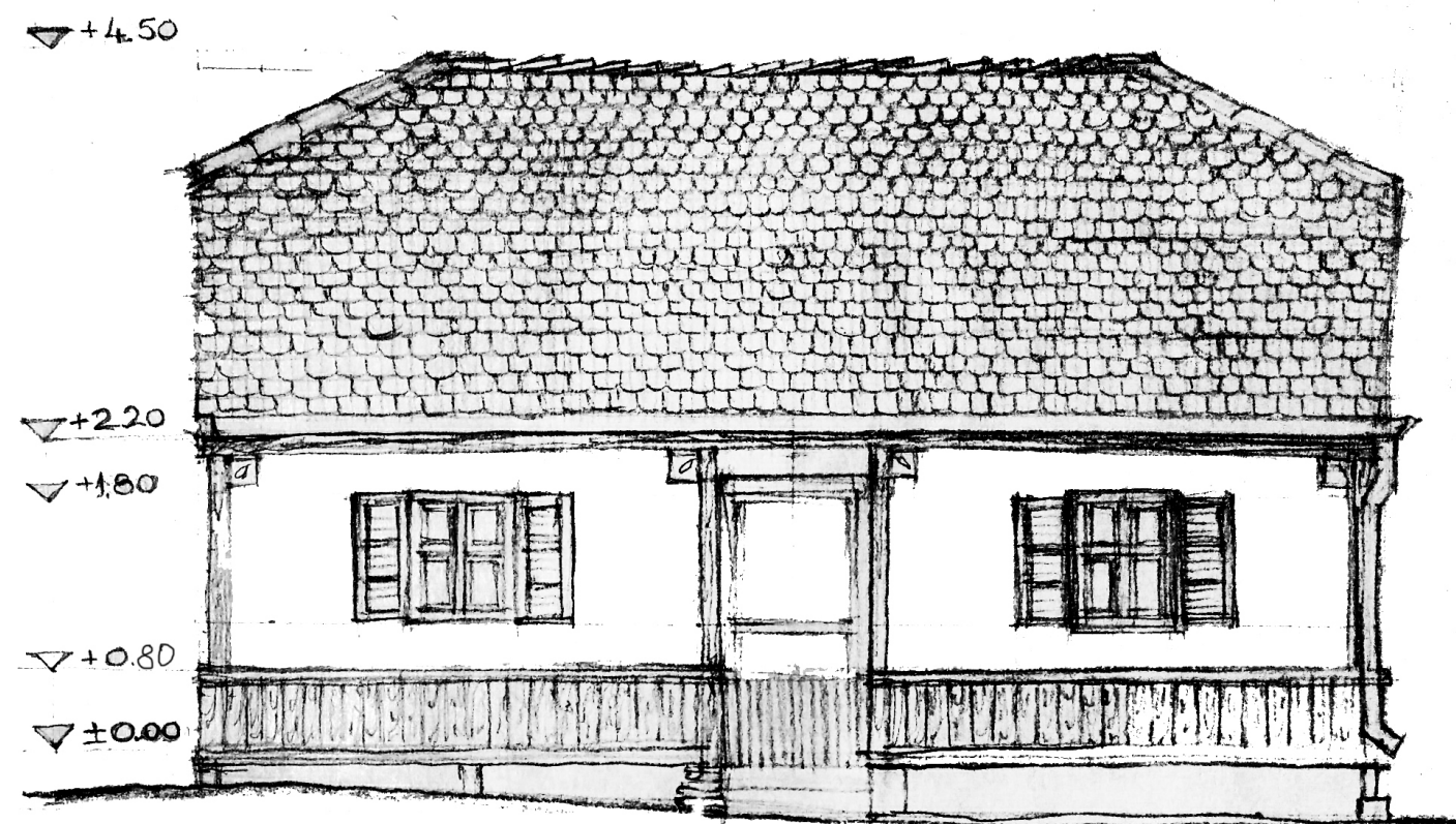
FATADA PRINCIPALĂ
