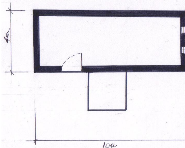
CRÎȘENI - CASĂ NR. 163 - PLAN PIVNITĂ
