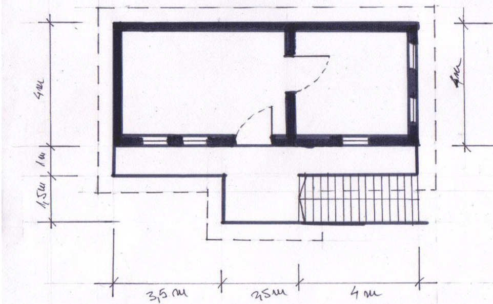
CRÎȘENI - CASĂ NR. 163 - PLAN PARTER
